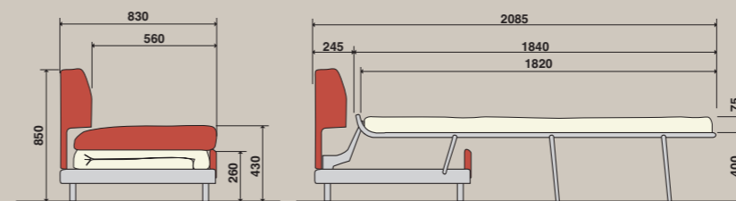
piede H 40/80
